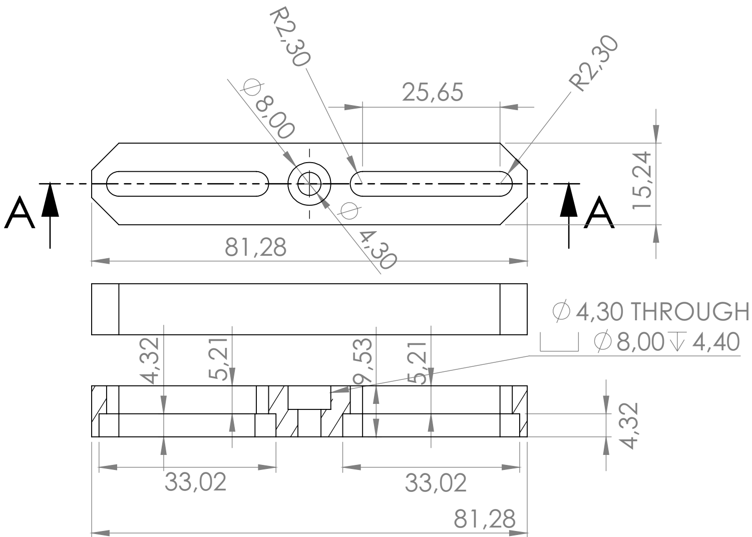
SECTION A-A
