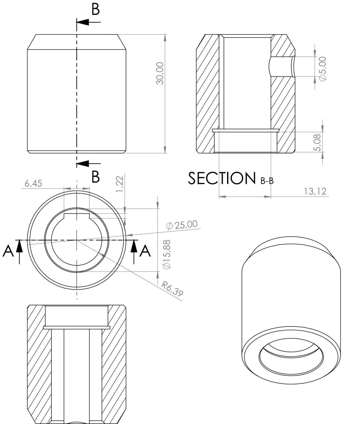
SECTION A-A
