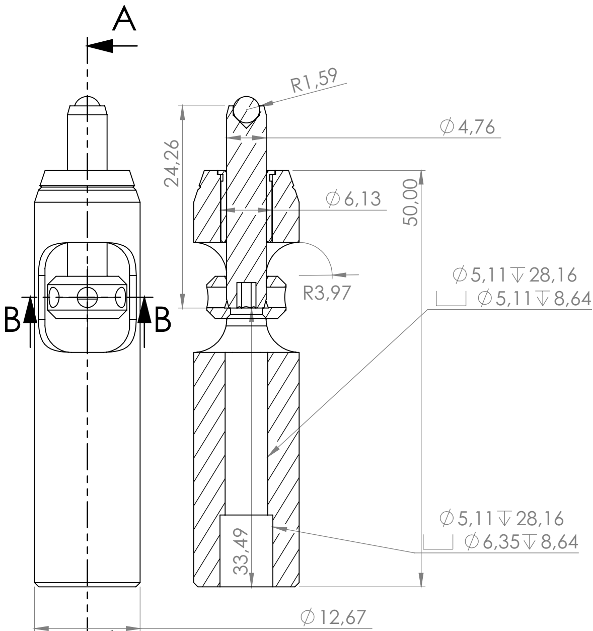
SECTION A-A
