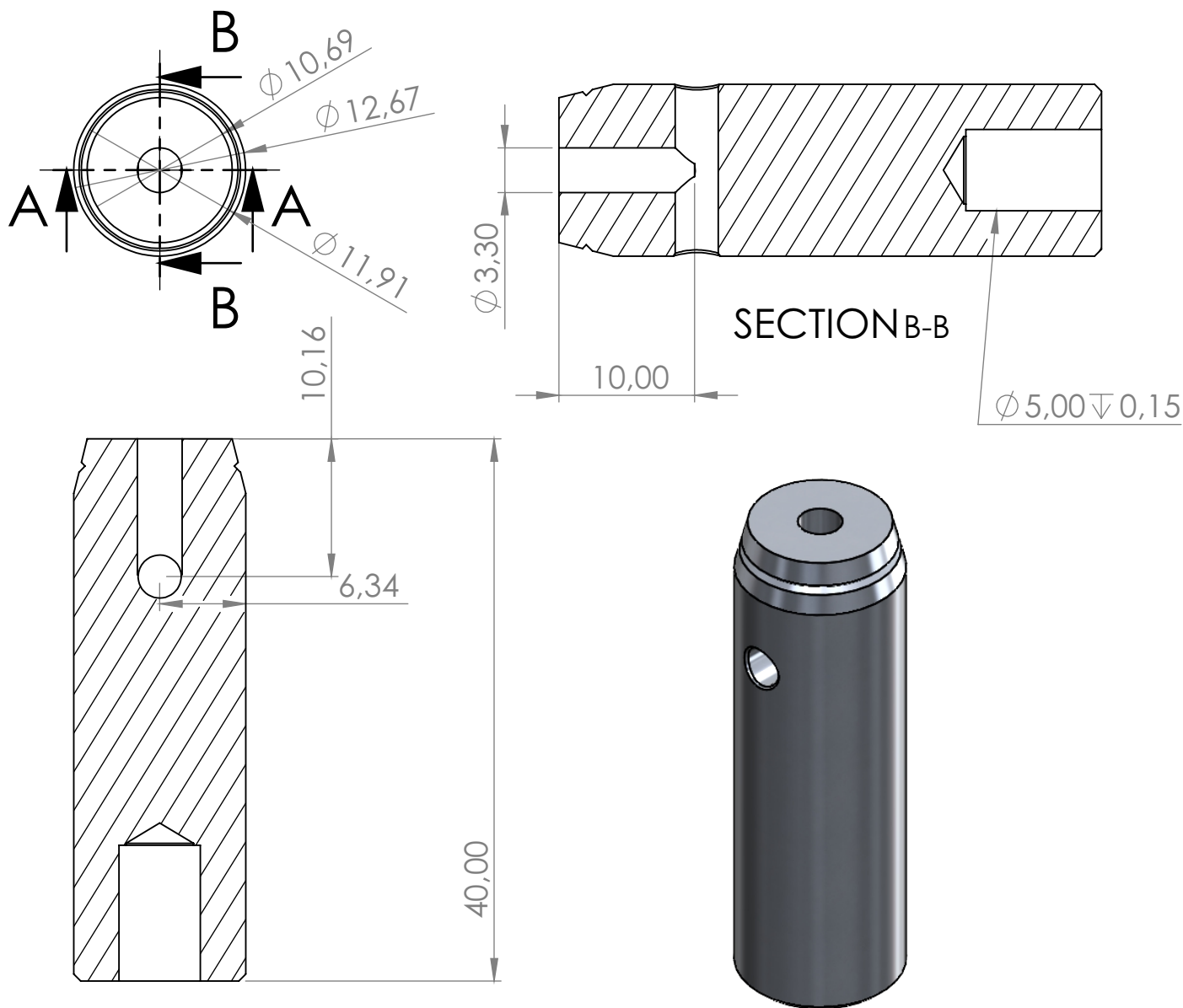
SECTION A-A
